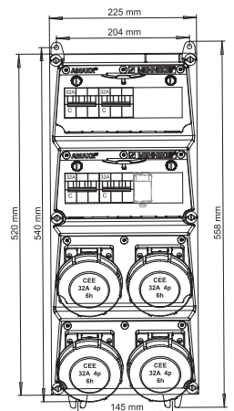
PLANO MECÁNICO
