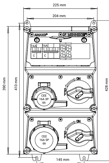
PLANO MECÁNICO
